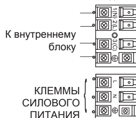
Клеммная колодка наружного блока
