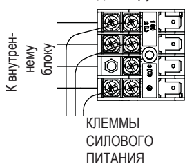
Клеммная колодка наружного блока
